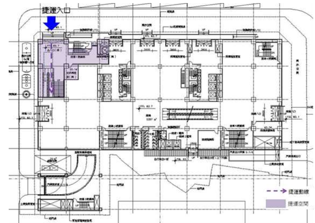
圖 2.2.3-1 地面層動線示意圖
