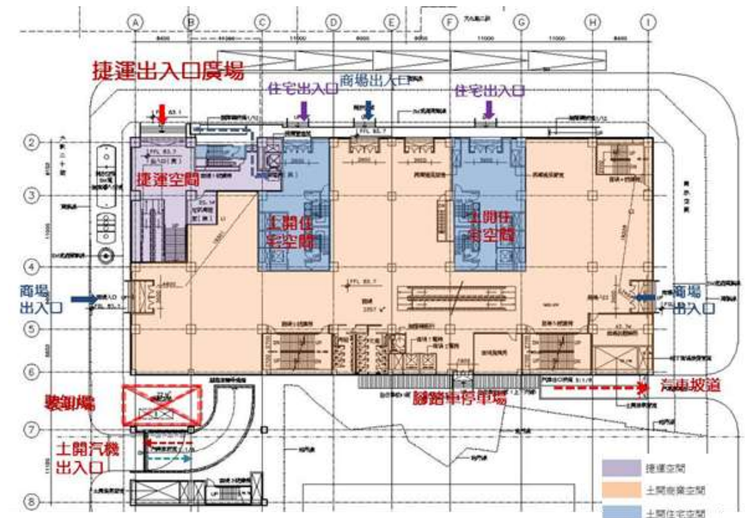
圖 2.2.3-5 地面層商場及住宅出入口動線示意圖
