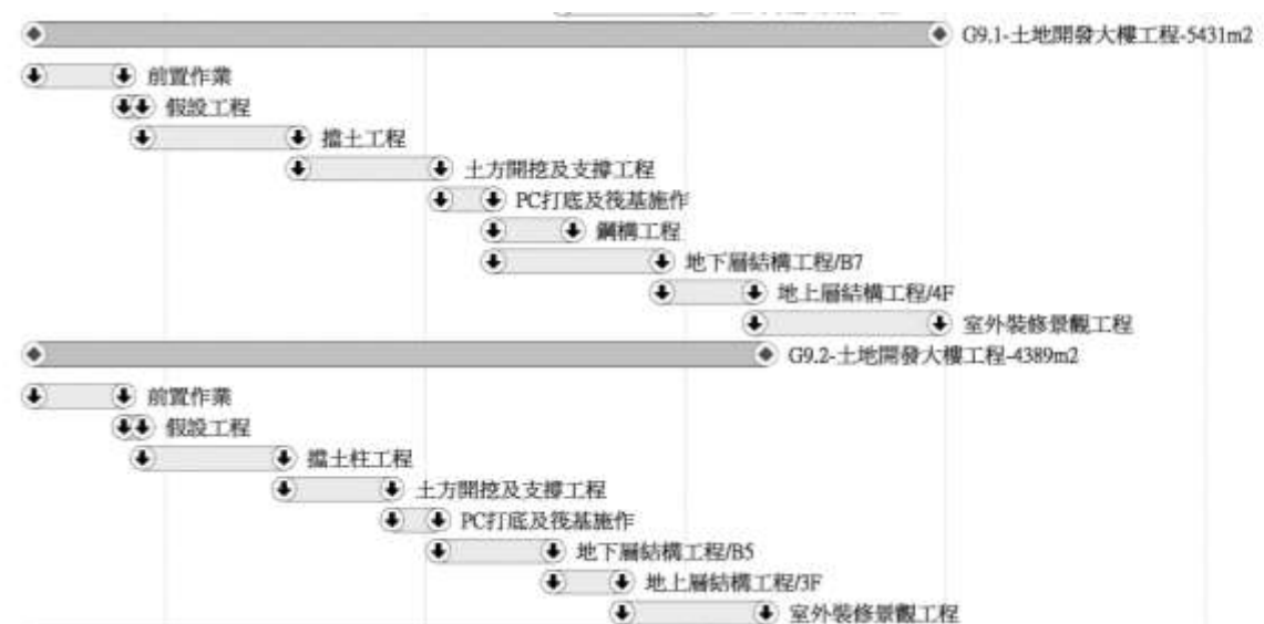
圖 5.2-1 G9-2 站工時程網狀圖
