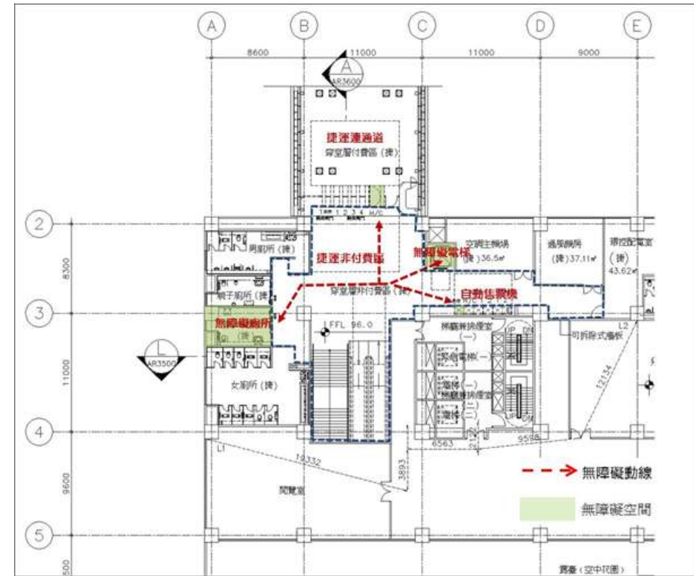
圖 2.2.5-2 三樓出層無障礙空間動線及配置圖
