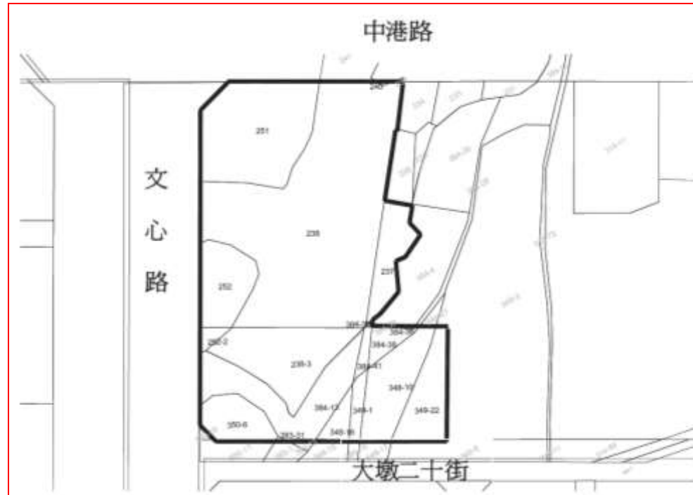
圖 1.2.2-1G9-2 地籍圖
