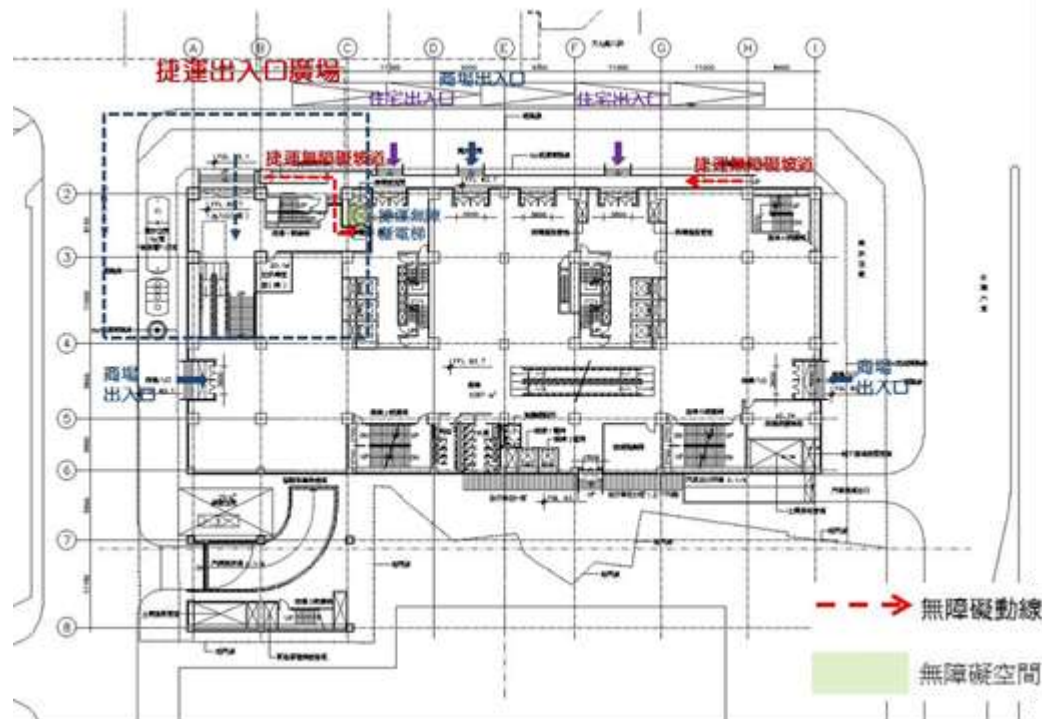
圖 2.2.5-1 一樓出入口無障礙空間動線圖
