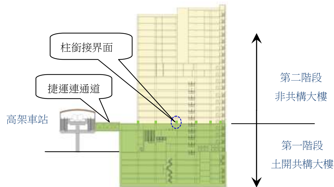
圖 3.2.2-1 捷運共構大樓分段施作示意圖
