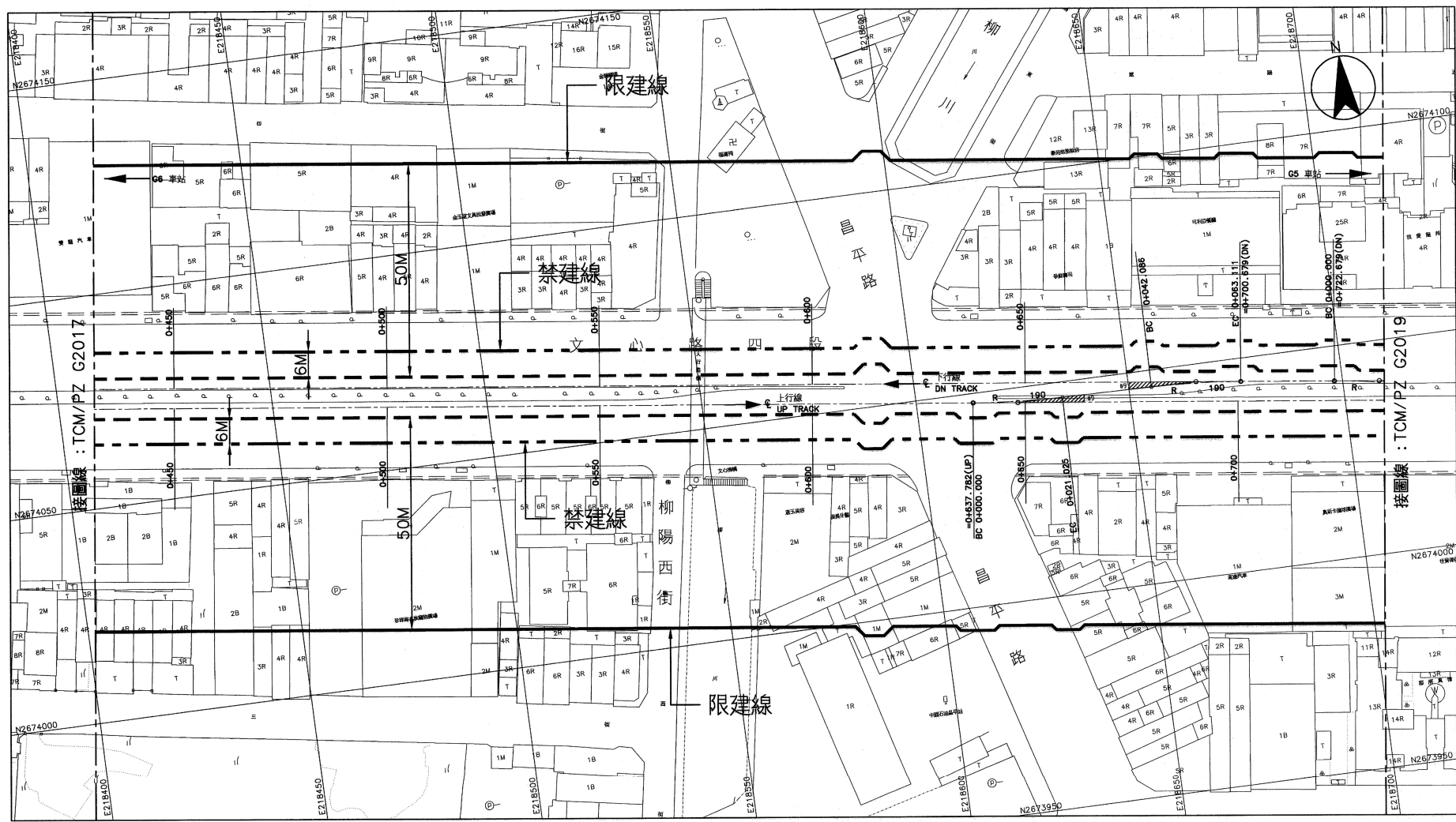
平面圖
