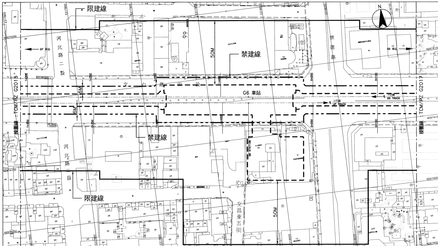
平面圖
