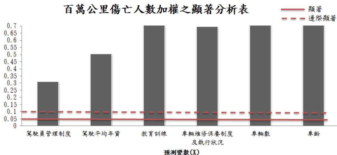
圖 9.2-2 百萬公里傷亡人數加權之顯著分析圖表
