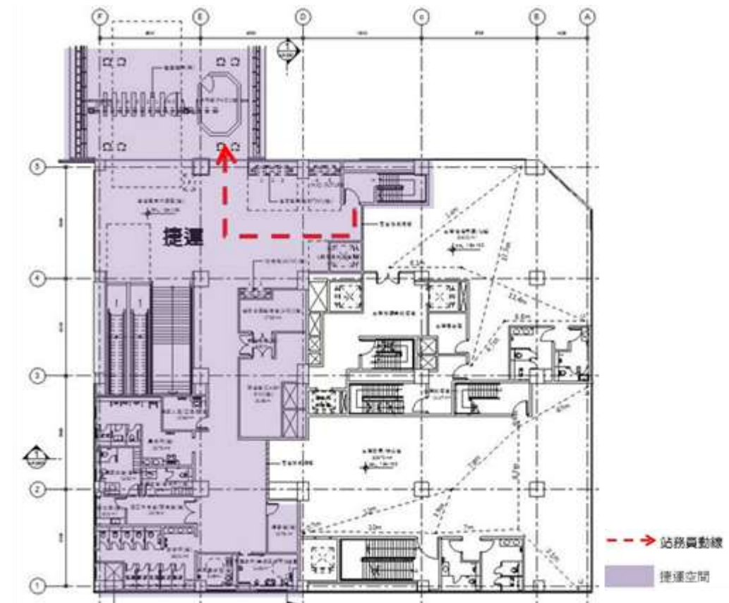
圖 2.2.3-6 三樓穿堂層動線示意圖
