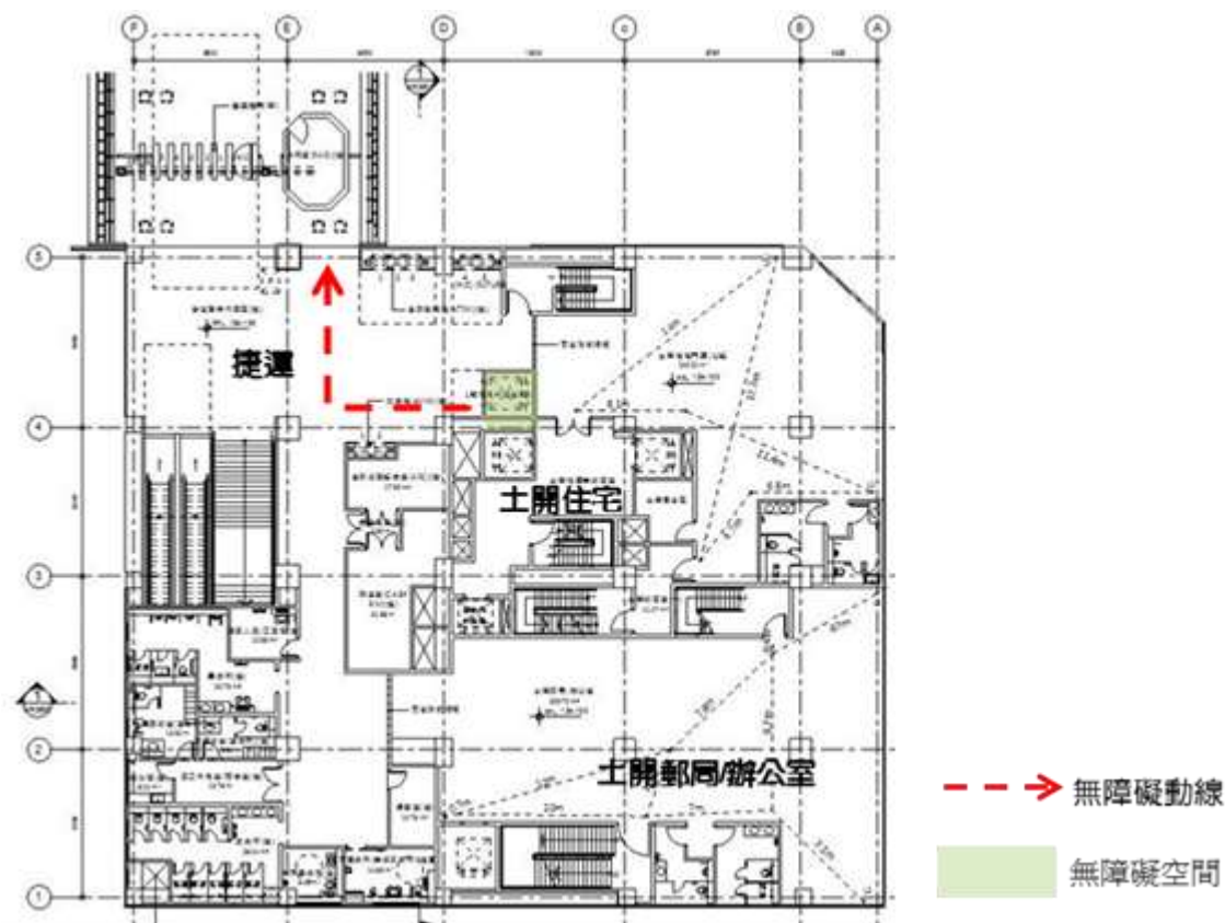
圖 9.2.5-2 三樓穿堂層無障礙空間動線及配置圖
