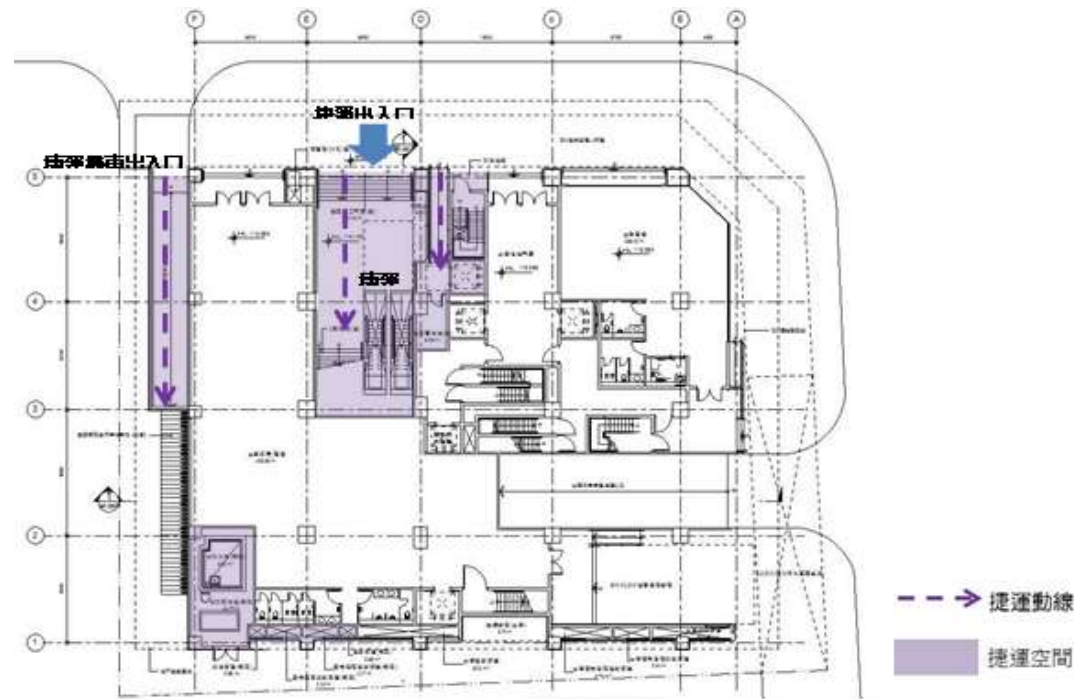
圖 2.2.3-1 一樓出入口動線示意圖
