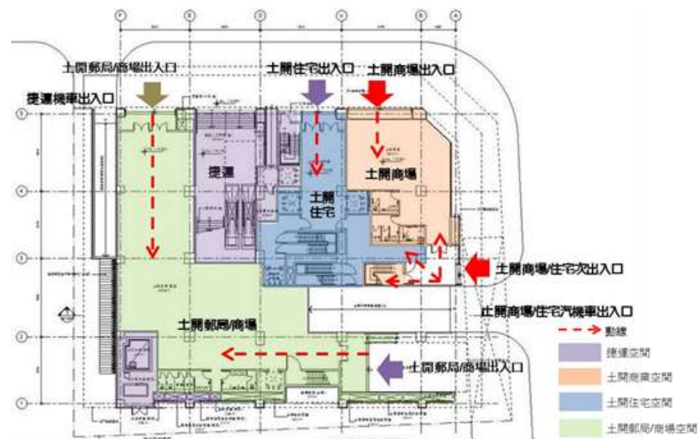
圖 2.2.3-7 一樓出入口動線示意圖
