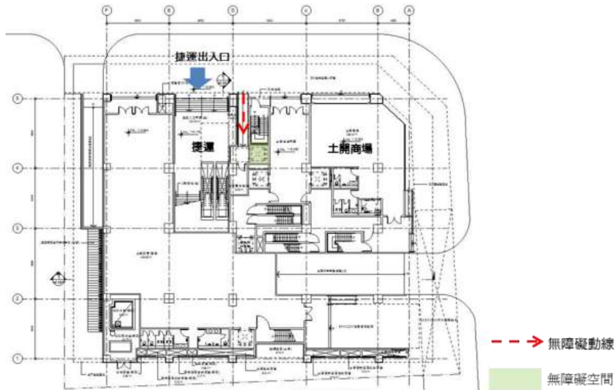
圖 2.2.5-1 一樓出入口無障礙空間動線圖
