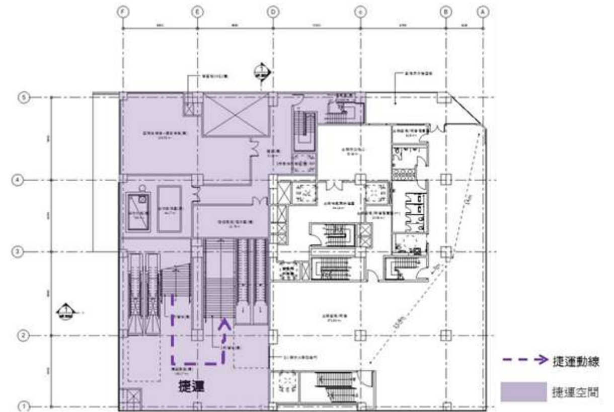
圖 2.2.3-2 二樓設備層動線示意圖
