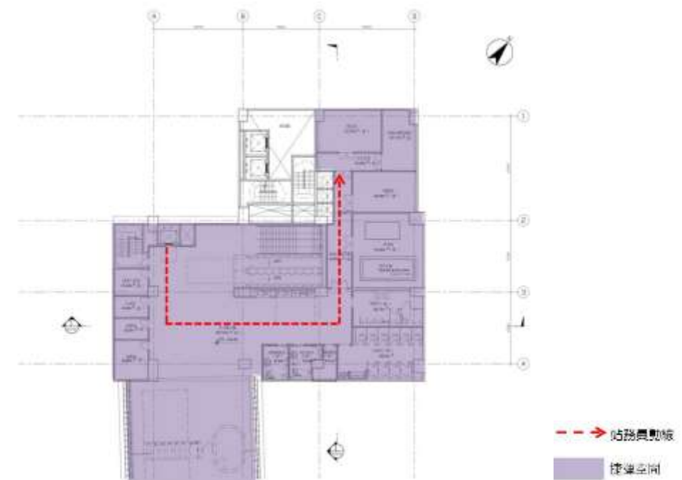
圖 2.2.3-6 三樓穿堂層動線示意圖
