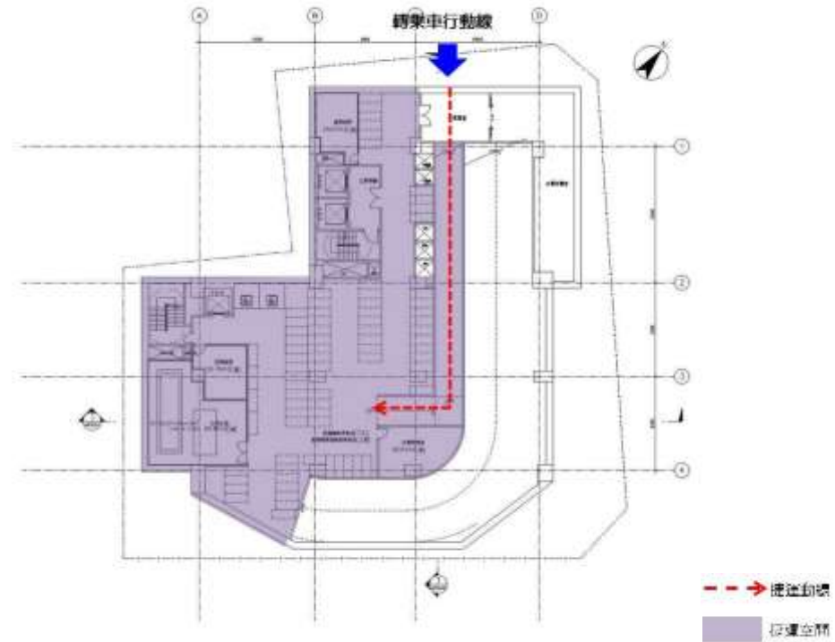
圖 2.2.3-4 地下一樓出入口動線示意圖
