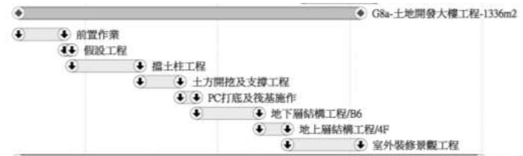
圖 5.2-1 G8a 站土開大樓施工時程網狀圖
