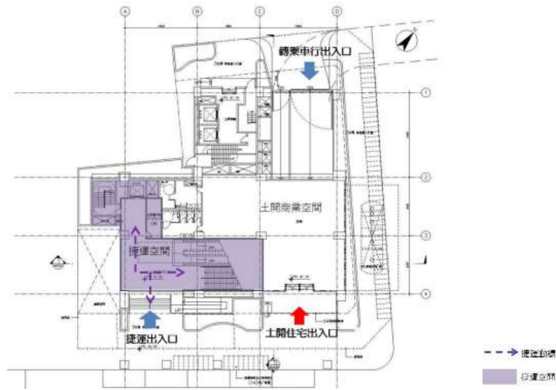
圖 2.2.3-1 一樓出入口動線示意圖
