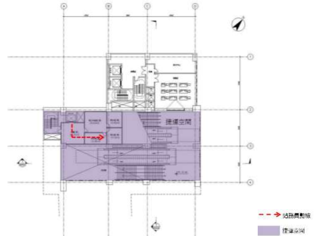
圖 2.2.3-5 二樓站務層動線示意圖
