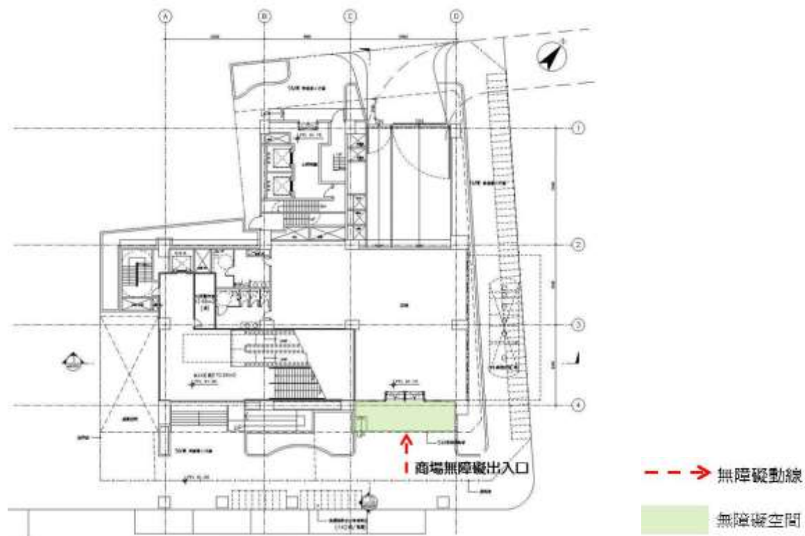
圖 9.2.5-4 地面層無障礙空間規劃示意圖
